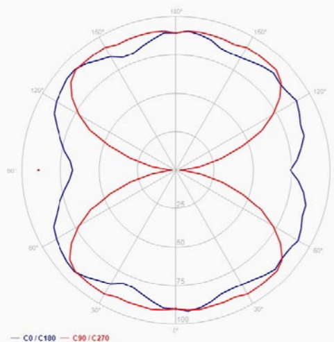
PHOTOMETRIC DIAGRAM, HUGO. DIAGRAMMA FOTOMETRICO DELLA HUGO.
